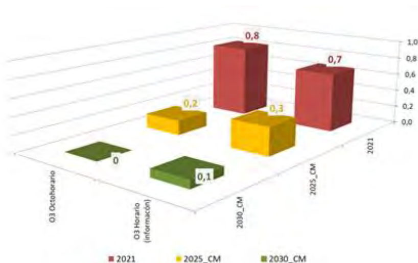
Figura 69. Porcentaje de área afectada por incumplimientos de valores límite/objetivo/umbral de los distintos contaminantes analizados para el año de referencia 2021 (modelo corregido) y los escenarios de emisiones de 2025 y 2030
