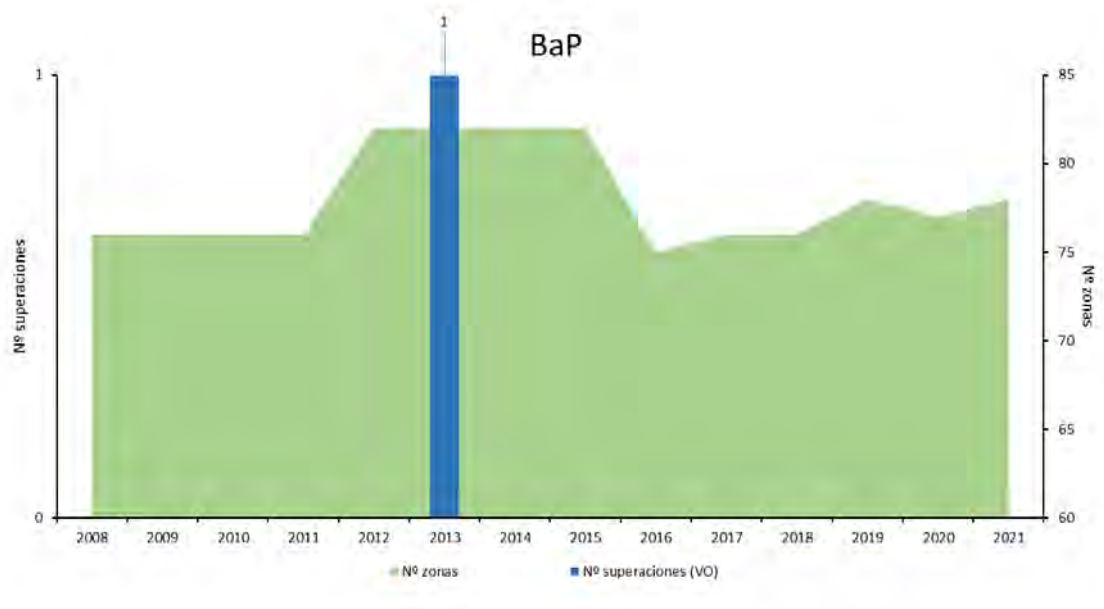
Figura 22. Número de superaciones de B(a)P (2008-2021)
