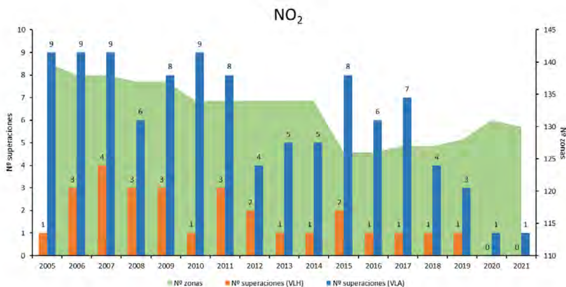
Figura 15. Número de superaciones de NO 2 (2005-2021)
