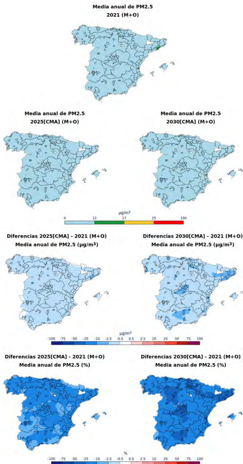
Figura 94. Concentración media anual de PM2,5 en 2021 (figura superior), concentraciones medias anuales estimadas para los escenarios CMA 2025 y 2030 (segunda fila), diferencias entre las estimaciones para 2025 y 2030 y las de 2021 (tercera fila) y diferencias relativas entre las estimaciones para 2025 y 2030 y las de 2021 (cuarta fila)
