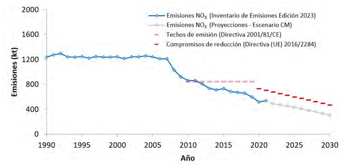
Figura 46. Evolución temporal de las emisiones de NO x computables según Directiva de Techos, desde 1990 hasta 2021, proyecciones del escenario CM hasta 2030 y relación con los techos de emisión y compromisos de reducción.
