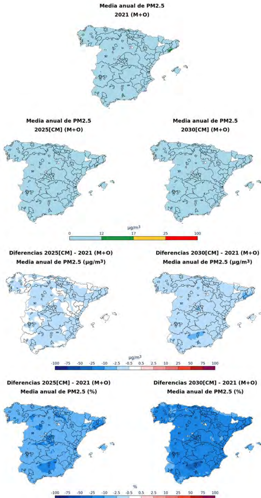
Figura 67. Concentraciones de PM 2,5 en 2021 (figura superior), y en los escenarios CM 2025 y 2030 (segunda fila). Diferencias entre las estimaciones para 2025 y 2030 y las de 2021 (tercera fila) y diferencias relativas entre las estimaciones para 2025 y 2030 y las de 2021 (cuarta fila)
