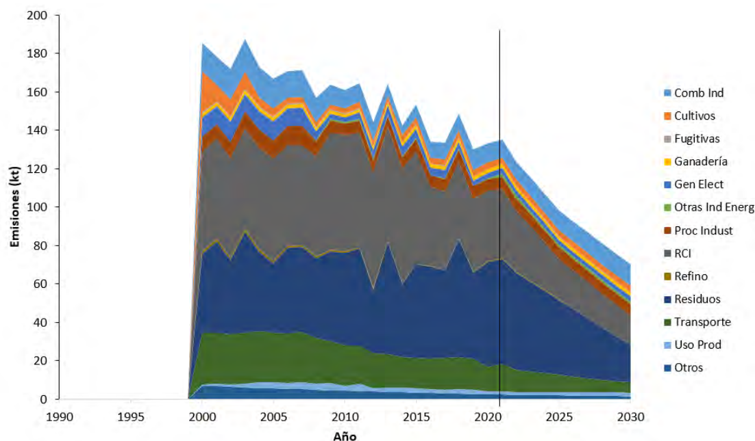
Figura 82. Emisiones de PM 2,5 según inventario (serie 2000-2021) y proyecciones (serie 2021-2030) bajo el escenario con medidas adicionales (CMA) desagregado para los principales sectores de actividad.
