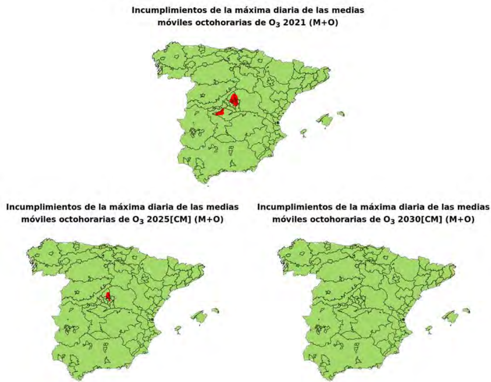
Figura 59. Las zonas en rojo indican las celdas en las que la modelización corregida estima incumplimientos de la normativa europea respecto al valor objetivo de O 3 con las emisiones 2021 (figura superior), y con las emisiones previstas para 2025 y 2030 (fila inferior).
