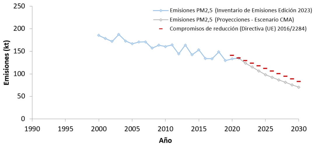
Figura 81. Evolución temporal de las emisiones de PM2,5 reportadas a Directiva de Techos desde 2000 hasta 2021, proyecciones del escenario CMA hasta 2030 y compromisos de reducción.
