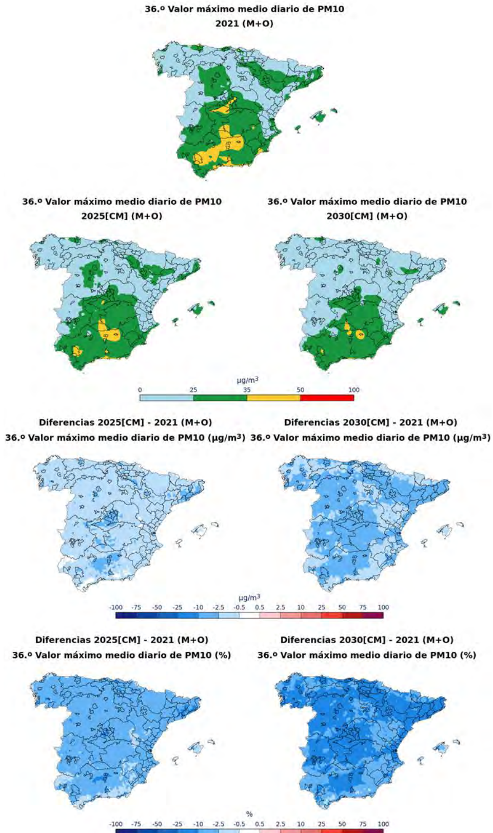
Figura 66. Concentración 36ª máxima diaria de PM10 en 2021 (figura superior), y en los escenarios CM 2025 y 2030 (segunda fila). Diferencias entre las estimaciones para 2025 y 2030 y las de 2021 (tercera fila) y diferencias relativas entre las estimaciones para 2025 y 2030 y las de 2021 (cuarta fila)
