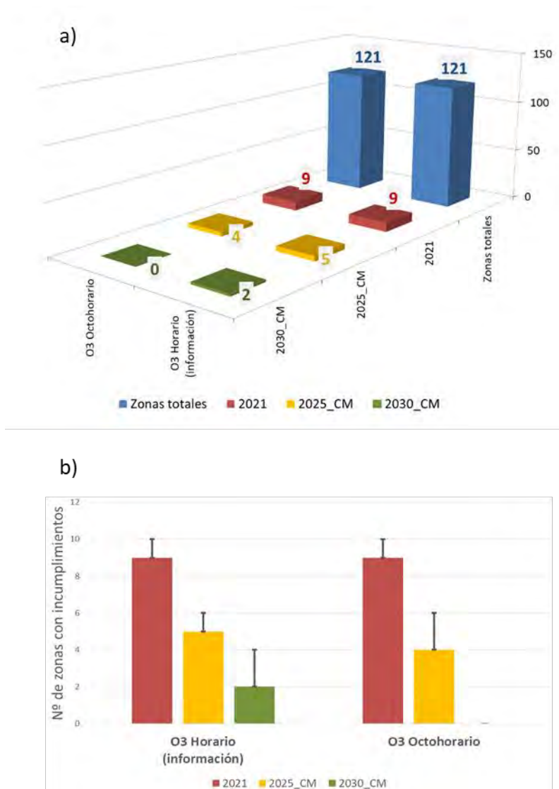
Figura 68. a) Número de zonas afectadas en la Península Ibérica y Baleares con incumplimientos de valores límite/objetivo/umbral de los distintos contaminantes analizados para el año de referencia 2021 (modelo corregido) y los escenarios de emisiones de 2025 y 2030. b) Rango de incertidumbre del número de zonas con incumplimiento, atendiendo al método de asignación de una celda a una zona de calidad del aire. (Nota: se muestran únicamente los contaminantes con problemas de incumplimiento)
