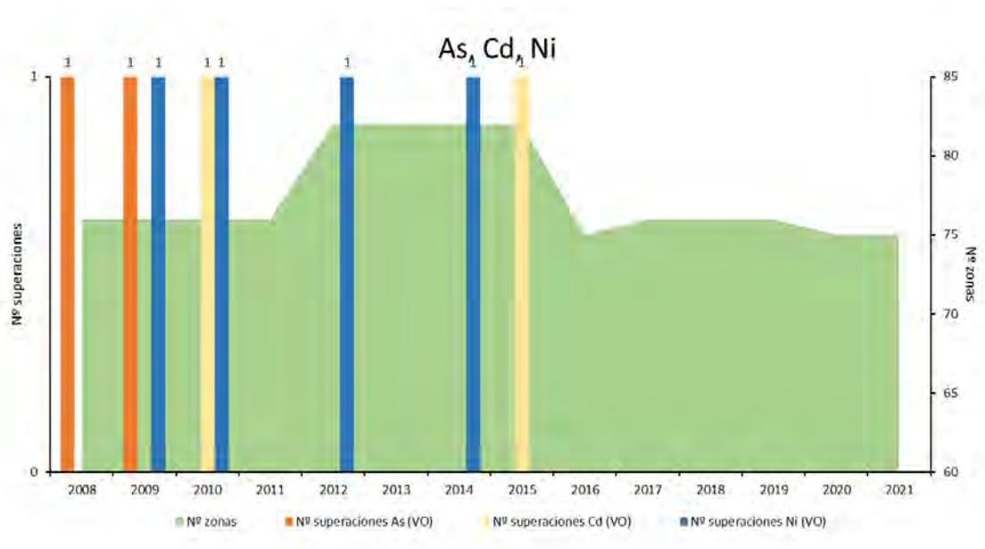
Figura 21. Número de superaciones de As, Cd, Ni (2008-2021)
